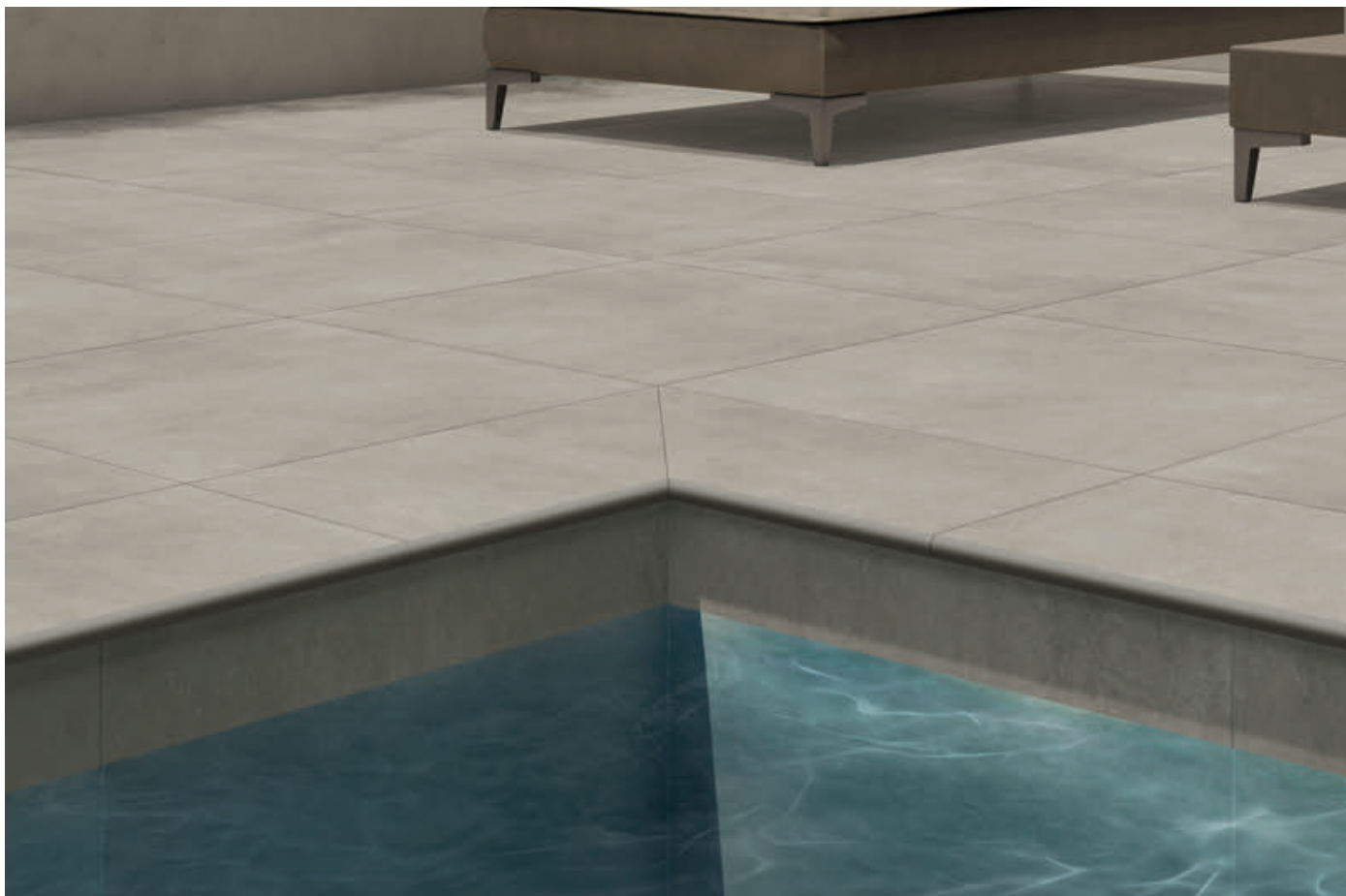
Randplatte gerundet mit Tropfkante · Border tile, rounded, with drip edge
