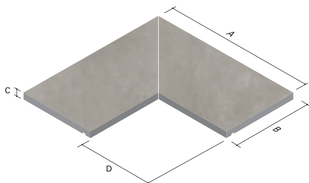
Randplatte mit Tropfkante – Innenecke (2-teilig) Border tile with drip edge - inside corner (2 pieces)
