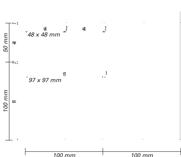
Kombination von Fliesen Nennmaß 5 x 5 cm, Kaliber 8 mit Fliesen Nennmaß 10 x 10 cm, Kaliber 7
