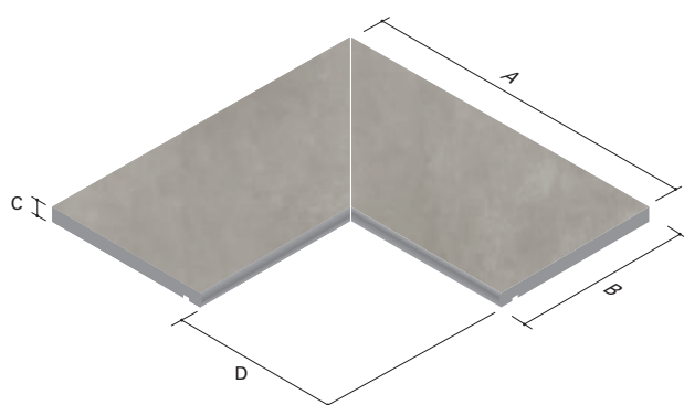
Randplatte gerundet mit Tropfkante – Innenecke (2-teilig) Border tile, rounded, with drip edge - inside corner (2 pieces)
