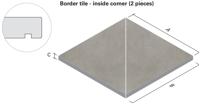
Randplatte – Innenecke (2-teilig) Border tile - inside corner (2 pieces)
